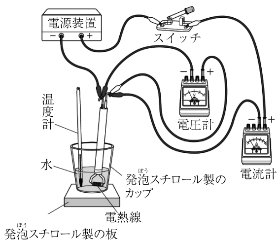
図 1 実験の装置図
